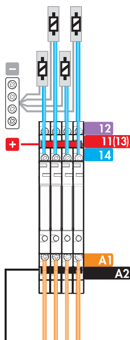
PLC - Saída
